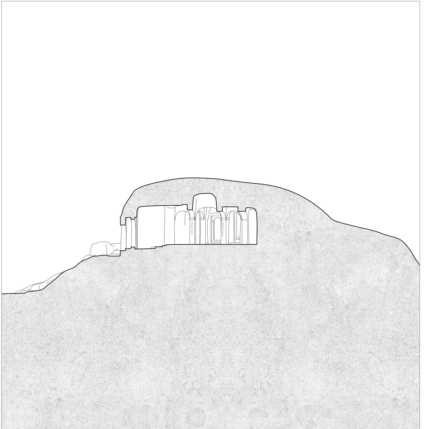
Däbrä Kidanä Mehrät Degum Section CC (2017)
