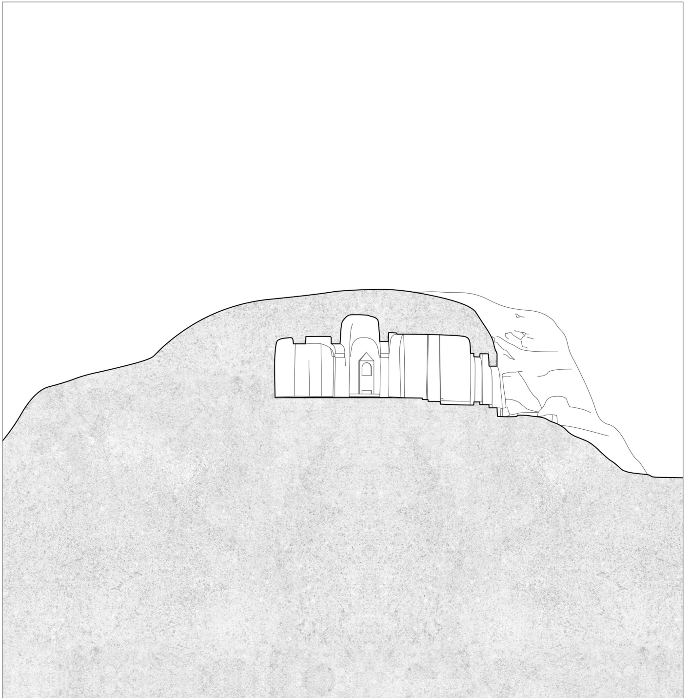
Däbrä Kidanä Mehrät Degum Section BB (2017)
